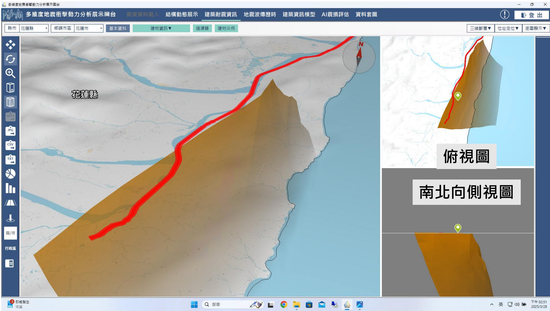
活動斷層地下三維模型
